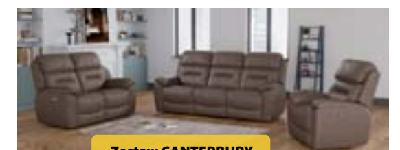
Zestaw CANTERBURY
